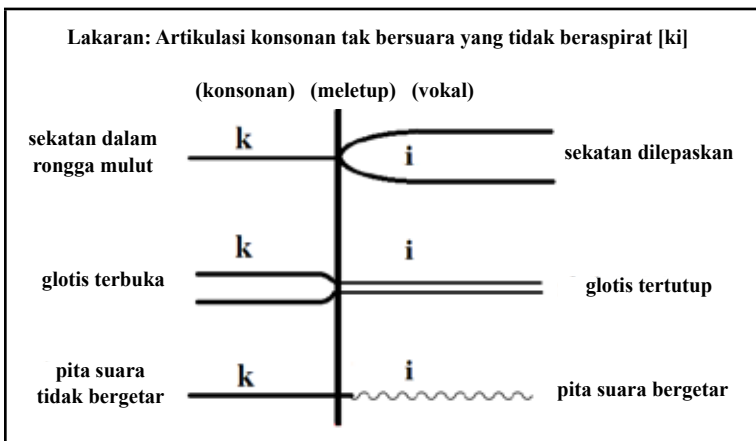
Rajah 6 Proses artikulasi gugusan bunyi [ki].
