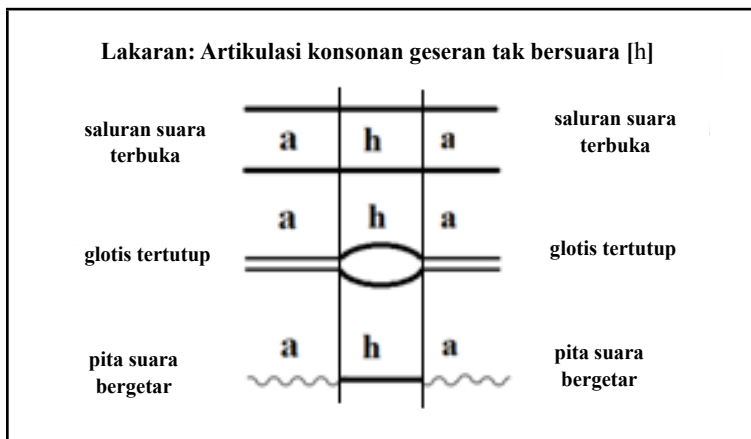
Rajah 14 Proses artikulasi gugusan bunyi aha [aha].
