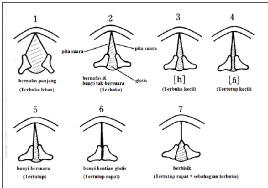
Rajah 1 Lakaran keluasan glotis dan pergerakan pita suara. 6 (Sumber: Tanaka et al. , 1987 hlm. 257)
