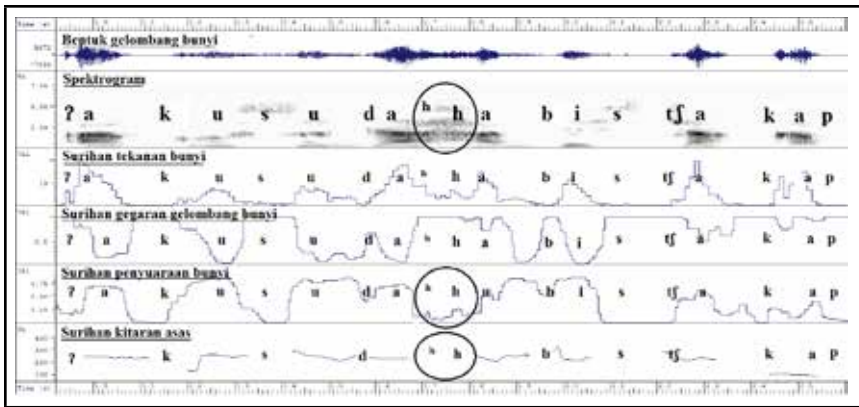
Rajah 2 Ayat Aku sudah habis cagak [ʔaku suda h habis tʃakap].
