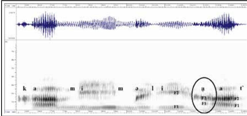
Rajah 12 Salinan vokal tak bersuara h [ə] dalam kata melihat [məliəat’].
