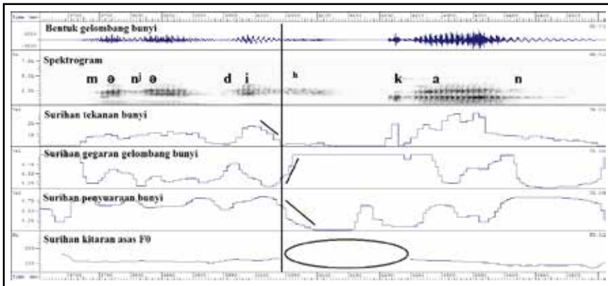
Rajah 11 Vokal beraspirat ih [i h ] dalam kata menyedihkan [məniədih h kan]. 13
