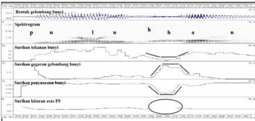
Rajah 21 Konsonan bergeminas h [ h h] dalam kata puluhan [pulu h han].
