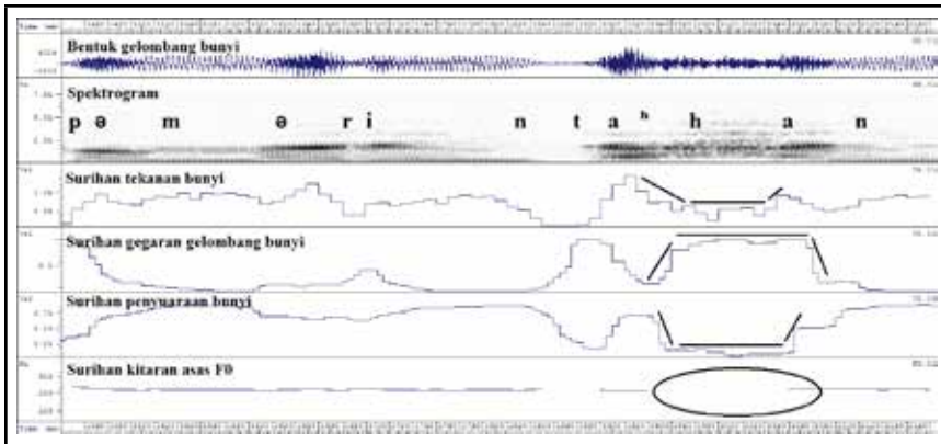
Rajah 27 Konsonan bergeminesi h [h h ] dalam kata pemerintahan [pəmərinta h hən].
