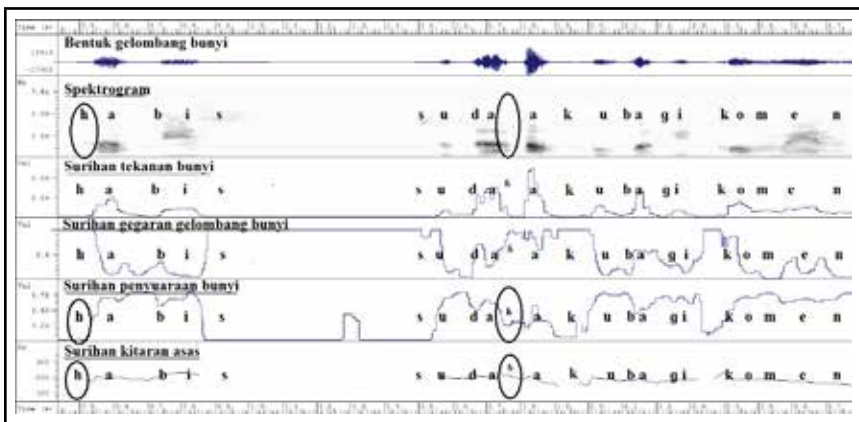
Rajah 3 Ayat Habis, sudah aku bagi komen [habis suda h aku bagi komen].
