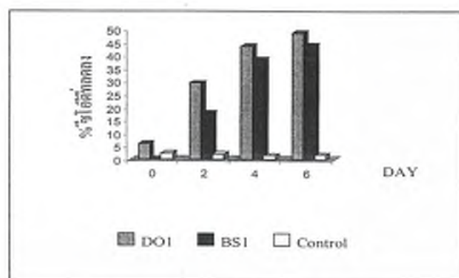
ภาพที่ 4 เปอร์เซ็นต์ซีโอดีที่ลดลงหลังจากทดสอบการบำบัดน้ำทิ้งจากโรงงานน้ำมันปาล์ม ด้วยเชื้อราหนร้อนที่คัดเลือกไว้ เป็นเวลา 6 วัน
