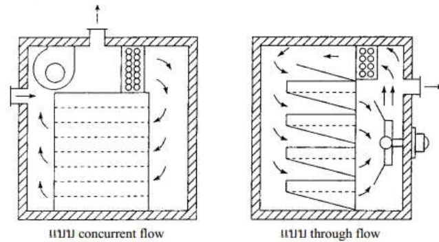
ภาพที่ 2.4 เครื่องอบ tray dryer ที่มา (Eng. Sut. ac. Th., 2558)
